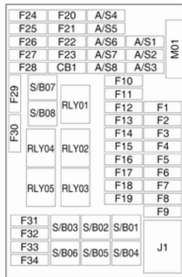
Минипредохранители
