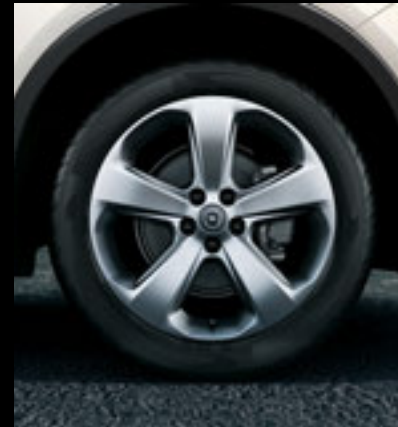
Leichtmetallrad 7 J x 18 im 5-Speichen-Design, Sterling Silver, Reifen 215/55 R 18 (RV6), Serie für Edition.
